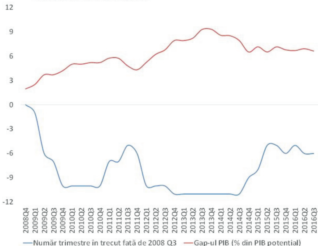
Fig. 1: Cel mai mare excedent de cerere (gap PIB pozitiv) înainte de 2009 a fost estimat pentru 2008 Q3 în runda de prognoză din 2008 Q4. Linia albastră arată că în toate estimările ulterioare, valorile cele mai apropiate de această valoare apăreau cu 8,3 trimestre mai devreme, arătând subestimarea sistematică a gap-ului PIB. Linia roșie arată valorile gap-ului PIB estimate pentru 2008 Q3 în rundele ulterioare de prognoză.
