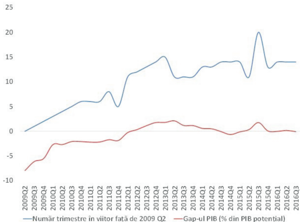
Fig. 2: Cel mai mare deficit de cerere (Gap PIB negativ) după 2008 a fost estimat pentru 2009 Q2 în runda de prognoză din 2009 Q2. Linia albastră arată că în toate estimările ulterioare, valorile cele mai apropiate de această valoare apăreau în medie cu 10,3 trimestre mai târziu, arătând supraestimarea gap-ului recesionist al PIB. Linia roșie arată valorile gap-ului PIB estimate pentru 2009 Q2 în rundele ulterioare de prognoză.
